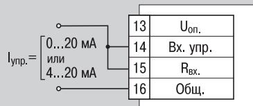
Ток 0...20 мА или 4...20 мА
