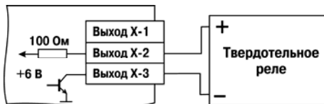
Рисунок Б.7 – Схема подключения нагрузки к ВУ типа Т
