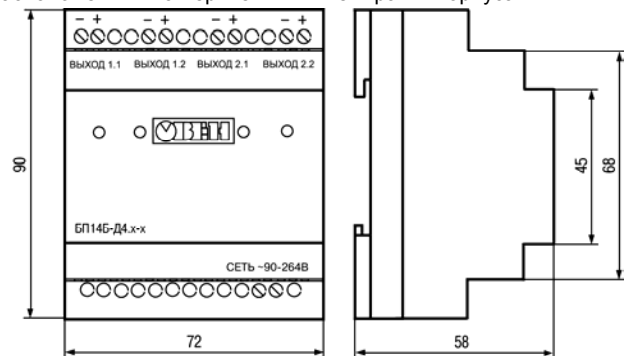
Рисунок 4.1 – Габаритные размеры блока питания БП14Б-Д4.х-хх
