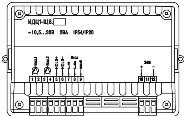
Рисунок 3.3 – Внешний вид задней панели прибора
