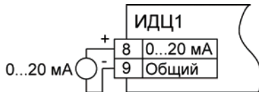
Рисунок 3.4 – Схема подключения ко входу прибора датчиков с сигналами тока от 0 до 5 мА, от 0 до 20 мА, от 4 до 20 мА
