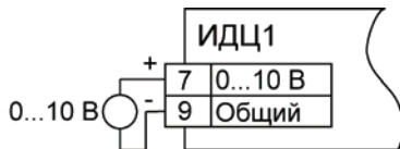
Рисунок 3.5 – Схема подключения к прибору датчиков с сигналами напряжения от 0 до 1 В, от 0 до 10 В
