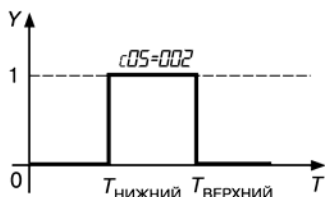
Рис. 3.16. Компаратор срабатывает внутри установленных пределов
