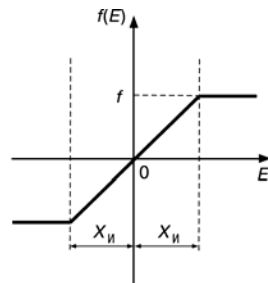
Рис. 3.9. Ограничение интегральной составляющей при помощи X_{н}
