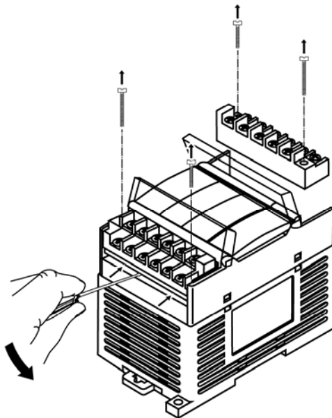
Рисунок Д.1 - Отделение съемных частей клемм МВ110
