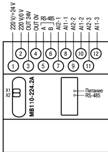
Рисунок Б.1 - Общий чертеж MB110-2A
