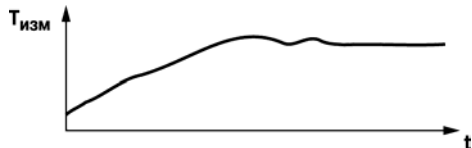
Рисунок 3.4, г - Включен фильтр in.FG и in.Fd
