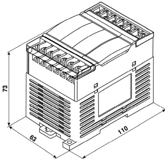
Рисунок А.1 - Габаритный чертеж MB110
