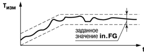
Рисунок 3.4, в - Включен фильтр in.FG
