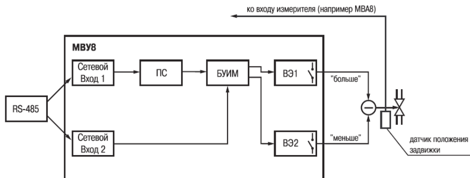
Рисунок 6.4 - Структурная схема управление трехпозиционным ИМ с датчиком положения
