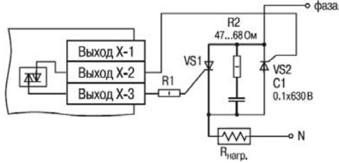
Рисунок Б.5 - Схема подключения к ВЭ типа С двух тиристоров, подключенных встречно-параллельно
