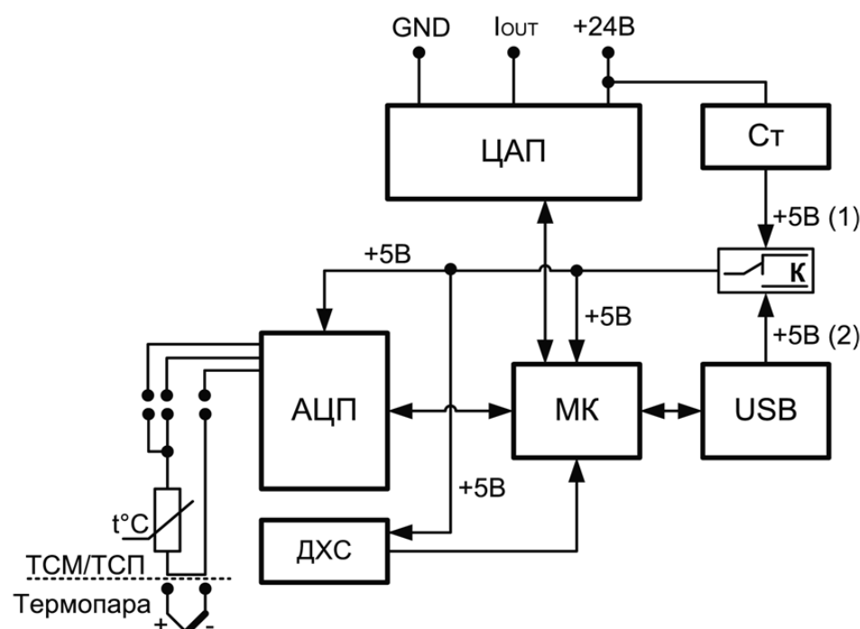
Рисунок 3.1 – Структурная схема преобразователя
