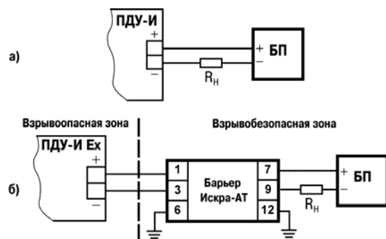
Рисунок Б.1 – Схема подключения датчика:
