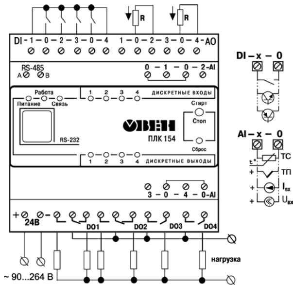
Рисунок Б.2 - Схема подключения питания, входов и выходов к ПЛК154-220.X-X
