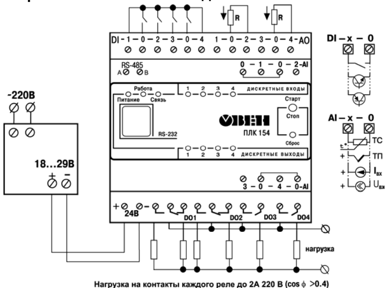
Рисунок Б.1 – Схема подключения питания, входов и выходов к ПЛК154-24.X-X
