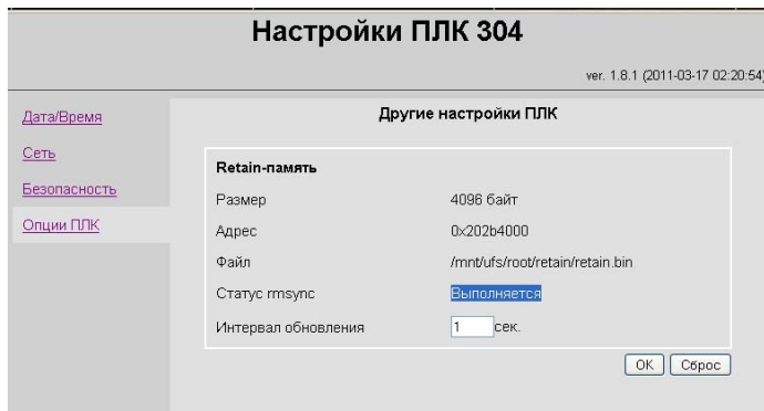
Рисунок Г.4 – Вкладка «Опции ПЛК304»
