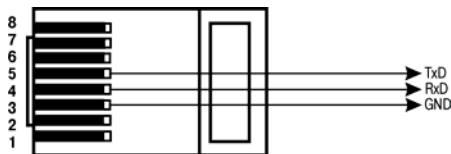
Рисунок Б.2 – Кабель связи ПЛК304 по RS-232 с внешним устройством
