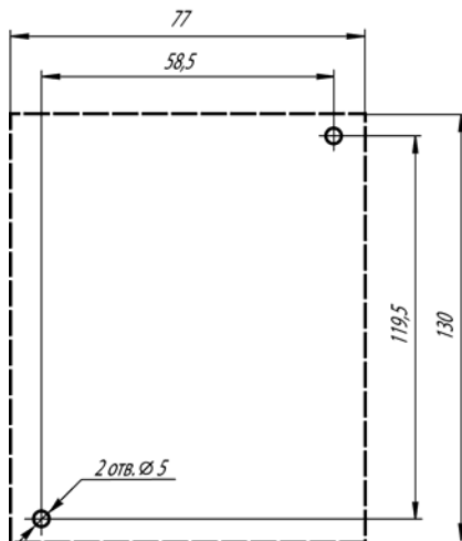
Рисунок А.2 – Разметка для установки на щит
