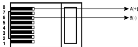
Рисунок Б.1 – Кабель связи ПЛК304 по RS-485 с внешним устройством
