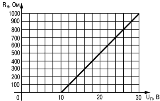
Рис 3.18. График зависимости R_n(U_n)
