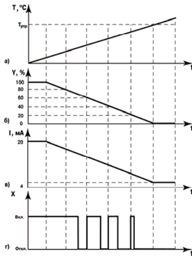
Рис. 3.11. Принцип управления в режиме “Нагреватель” а) изменение температуры объекта; б) сигнал на выходе регулятора; в) сигнал на аналоговом выходе типа I; г) сигнал на дискретном выходе типа P
