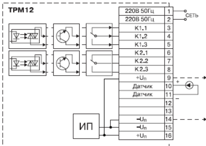
Рисунок Г.3 - Схема подключения к приборам TPM12X датчиков с унифицированными выходными сигналами тока и напряжения (для конструктивного исполнения "Н", "Щ1" и "Щ2")
