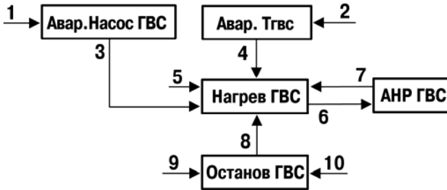
Рисунок 4.1 – Схема перехода между режимами контура ГСВ
