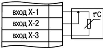
а) термопреобразователь сопротивления ТСМ/ТСП
