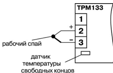
Рисунок 3.4 – Схема подключения ТП
