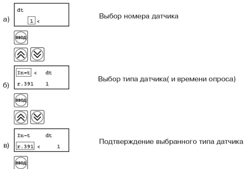
Рисунок 5.2 – Порядок настройки аналоговых входов (выбор номера, типа, значения параметра – производить кнопками и ; символ «<» обозначает изменяемое поле)
