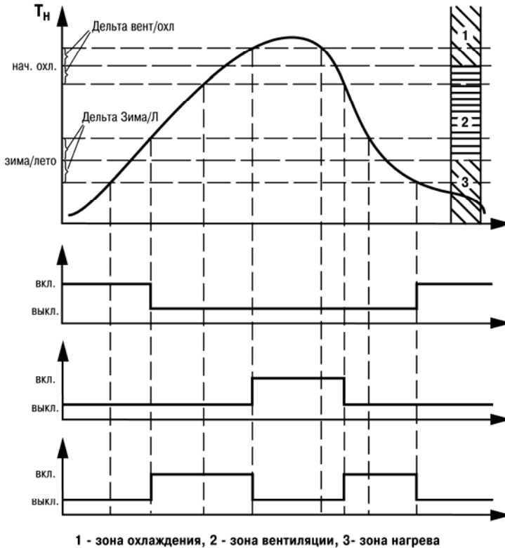
Рисунок 5.2 – Условия перехода между режимами «Нагрев»-«Вентиляц»-«Охлаждение»
