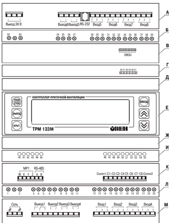
Рисунок 3.1 – Прибор ТРМ133М-02: внешние связи, элементы индикации и управления
