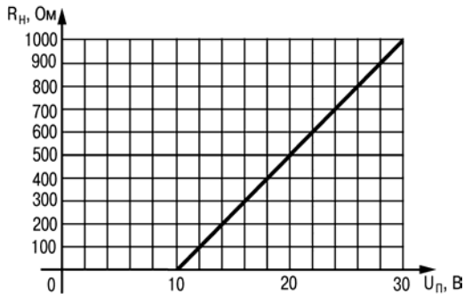
Рисунок 3.6 - График зависимости R н (U п )
