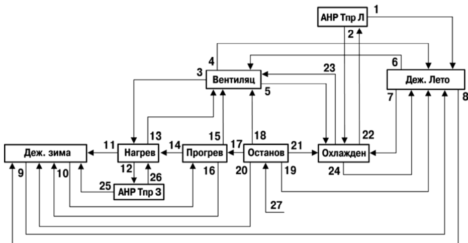
Рисунок 5.1 – Схема перехода между режимами
