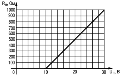
Рисунок 3.7 - График зависимости R н (U п )
