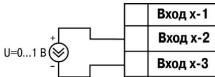
Рисунок Б.5 – Подключение активного датчика с выходом в виде напряжения 0...1 В
