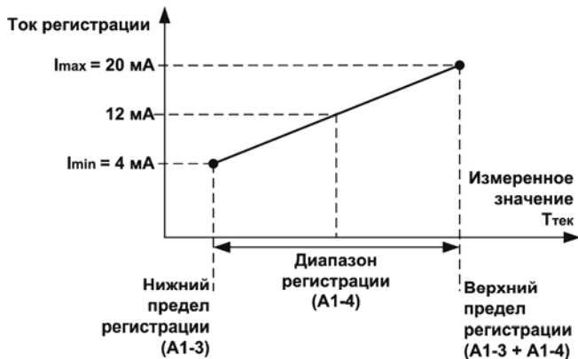
Рисунок 3.13 – Принцип формирования тока регистрации
