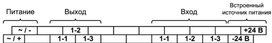
Рисунок Б.1 – Клеммная колодка прибора
