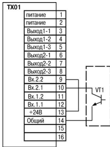
Рисунок Б.2 – Подключение пассивных датчиков, имеющих на выходе транзистор n-p-n типа с открытым коллекторным входом:
