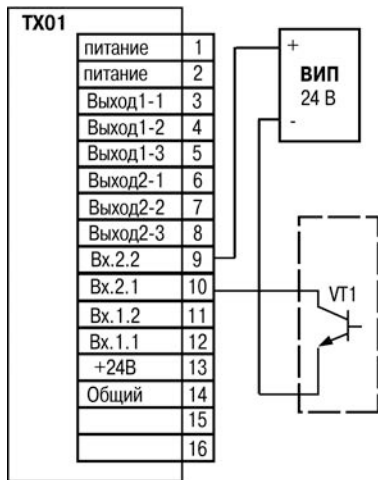
Рисунок Б.2 – Подключение пассивных датчиков, имеющих на выходе транзистор n-p-n типа с открытым коллекторным входом:
