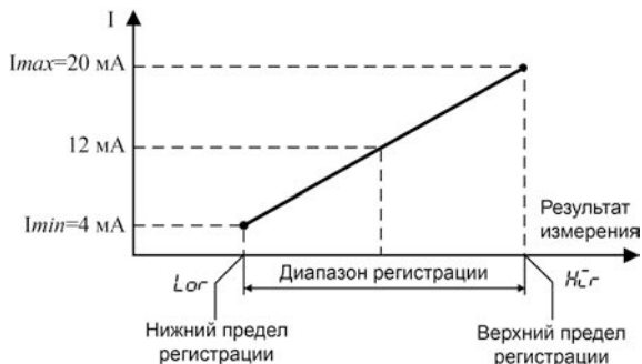
Рисунок 4.5 – Принцип формирования выходного сигнала ВУ в режиме регистратора для приборов с ВУ типа И
