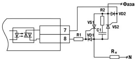
Рисунок Б.6 – Схема подключения к ВУ типа С двух тиристоров, подключенных встречно-параллельно
