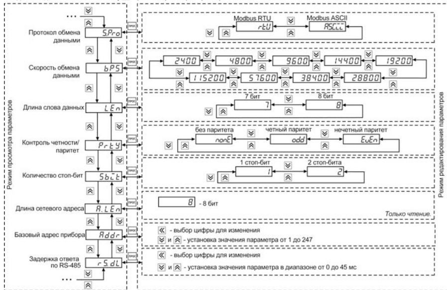
Рисунок 4.12 – Меню «Настройка параметров связи с ПК»
