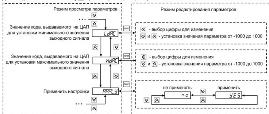
Рисунок 4.11 – Меню «Юстировка»
