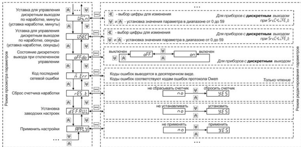
Рисунок 4.10 – Меню «Конфигурация» (окончание)
