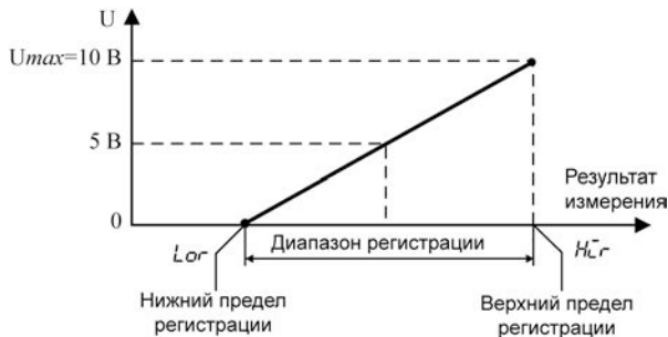
Рисунок 4.6 – Принцип формирования выходного сигнала ВУ в режиме регистратора для приборов с ВУ типа У
