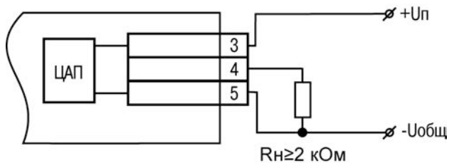
Рисунок Б.8 – Пример подключения ВУ типа У
