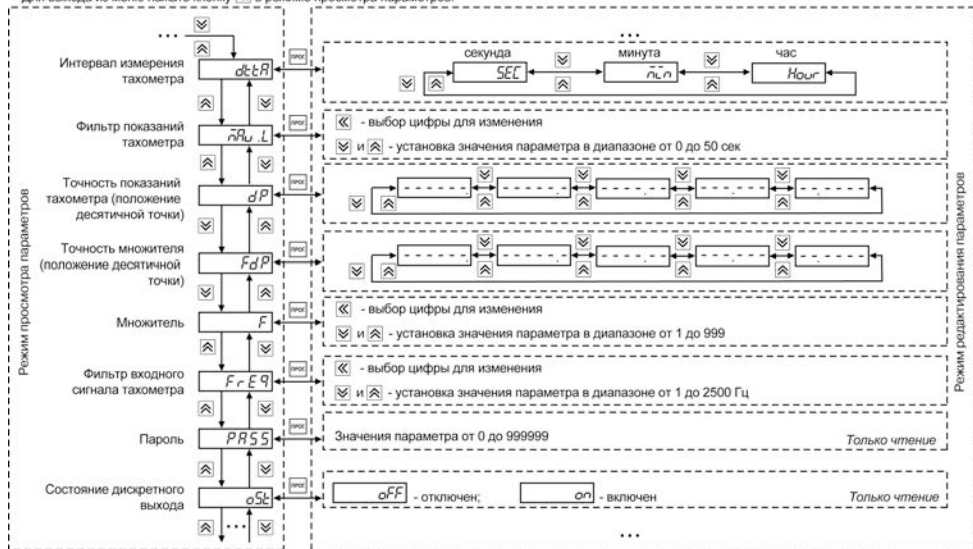
Рисунок 4.7 – Меню «Конфигурация»
