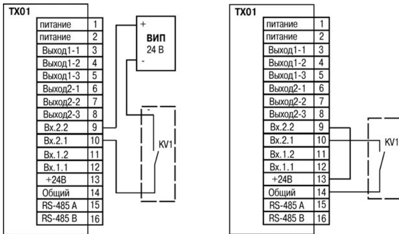
Рисунок Б.1 – Подключение к входу коммутационных устройств: а) при работе датчика от внешнего источника питания; б) при работе датчика от внутреннего источника питания
