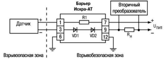
Рисунок 1 – Схема подключения барьера, R1=390 Ом ±5 %; VD1, VD2 – диоды КД208
