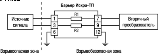
Рисунок 2 – Схема подключения барьера, R1=R2=110 Ом ±5 %
