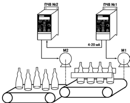
Рисунок 4.14 – Схема установки
