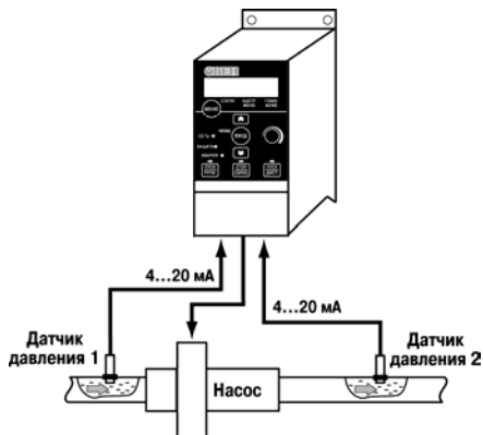
Рисунок 4.11 - Структурная схема установки
