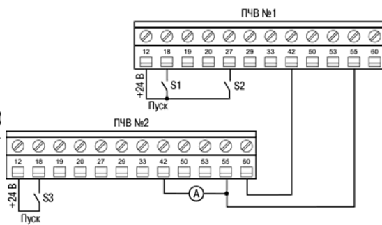
Рисунок 4.15 – Подключения ПЧВ №1 и ПЧВ №2
