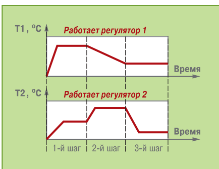
▲ Пример программы для двухканального регулятора TRM151-01
