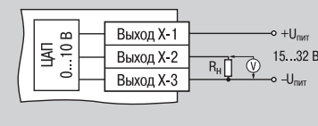
Выходной элемент типа У (ЦАП 0...10 В)
