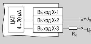
Выходной элемент типа И (ЦАП 4...20 мА)
